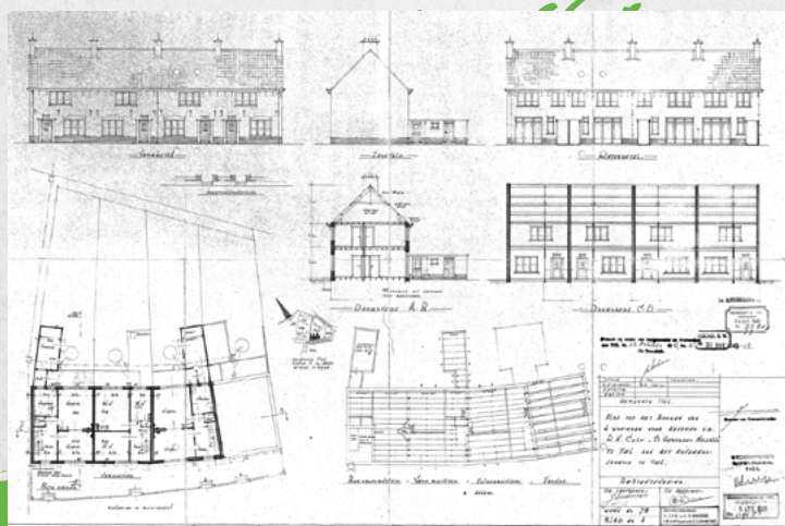
Bouwtekening voor het bouwen van 4 woningen aan het Hovenierslaantje in Tiel door R.K. Coöp. St. Gerardus Majella in 1946. Bron: RAR 1667-BL1946010.
